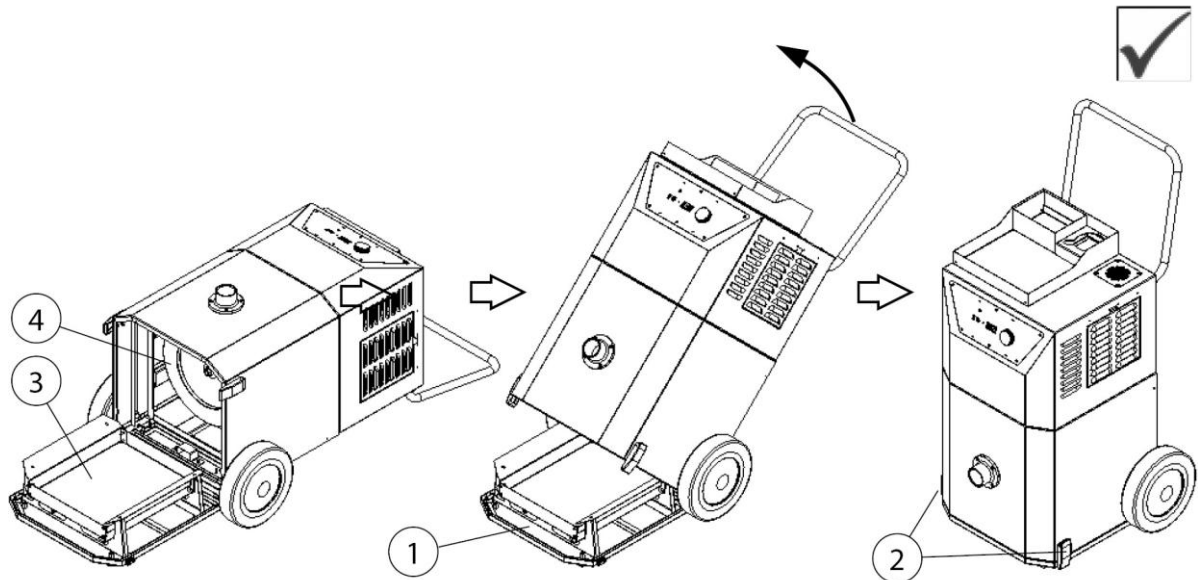
Abb. 13: Wartungsdeckel verschließen
